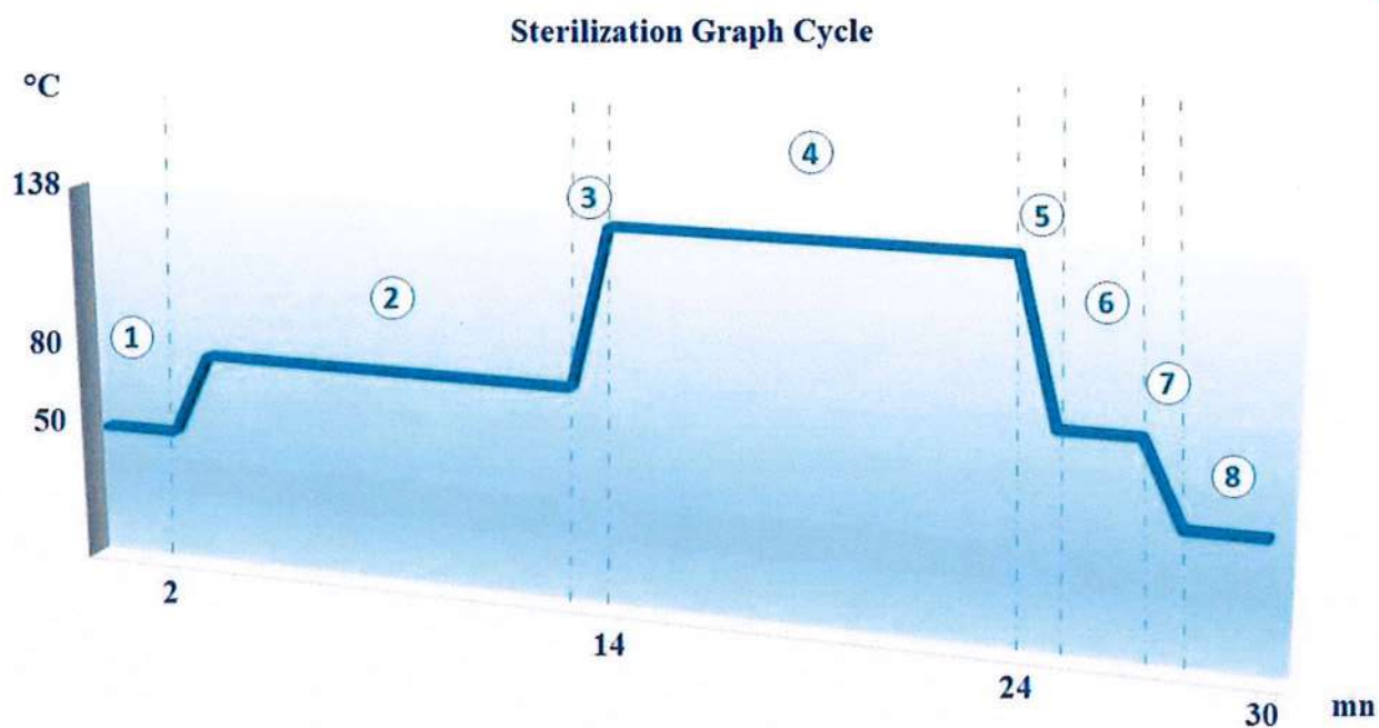
Figure 7. Paraqitja grafike e ciklit te sterilizimit.
